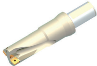
Е2. Усиленное сверло
