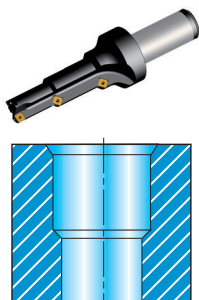
В4. Уступ и фаска
