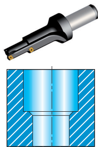
В5. Зенковка и фаска
