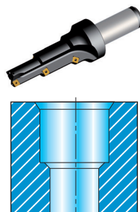
В6. Зенковка с фасками
