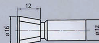
Fresa a profilo inclinato No. 033611
